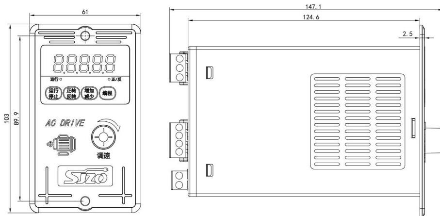
I/O-2控制
