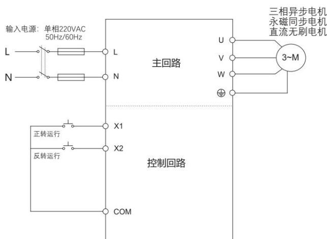
21Y系列接线原理图
